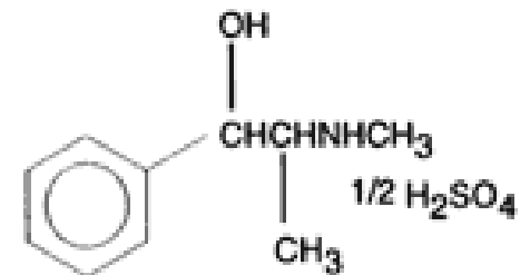
Efedrina
