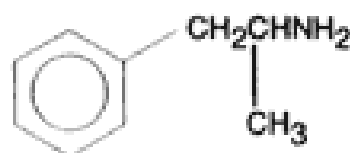
Anfetamina
