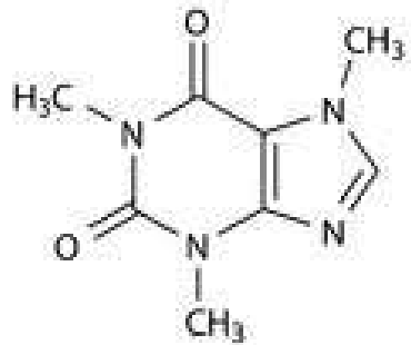
Caffeine
